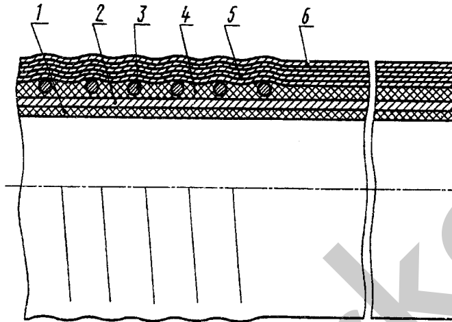
Схема конструкции рукава
